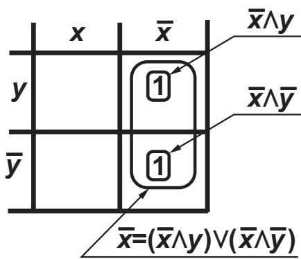
Рис. 3.6. Карта Карно
