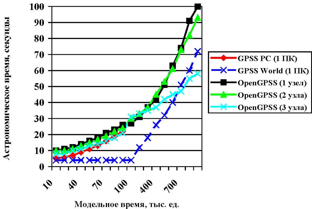
Рис.4. Сравнение скорости моделирования
